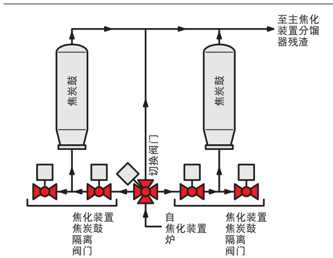
4通焦炭鼓切换阀门的主要功能是将进料流从一个焦炭鼓导向另一个焦炭鼓。
